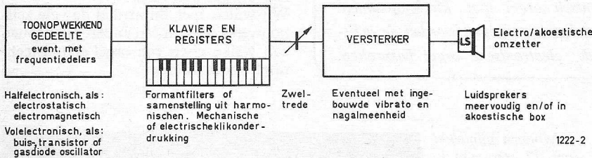
Figuur 3. Algemeen blokschema van elektronisch-orgel.
