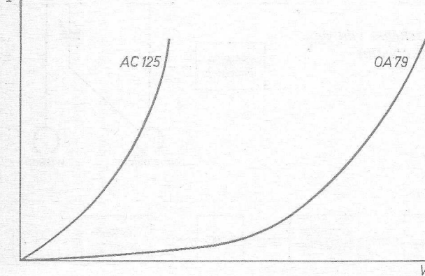
Figuur 4: Stroom/spannings-karakteristieken bij een als diode geschakelde transistor AC 125 en een germaniumdiode OA 79.
