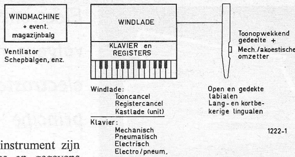
Figuur 2. Algemeen blokschema van een pijporgel.
