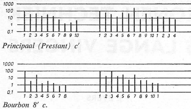
Figuur 9. Verschil in de boventonen tussen gelijksoortige stemmen van verschillende orgeltypen - boven een zuidoosts Silbermann-orgel en onder een Duitse orgel uit 1900.
