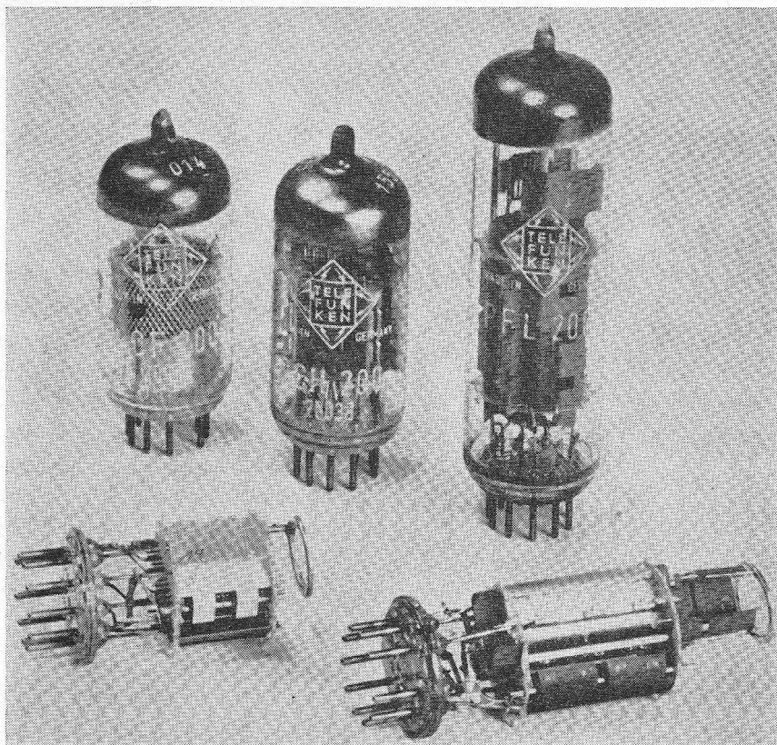
De nieuw-ontwikkelde 10-pens PCF200, PCH200, PFL200. Foto Telefunken.
