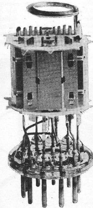
PCH200 de nieuw ontwikkelde 10-pens triode-heptode voor gebruik in sync-scheiders.
