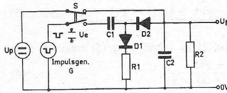
Figuur 1. Principe-schakeling van de diodepomp
