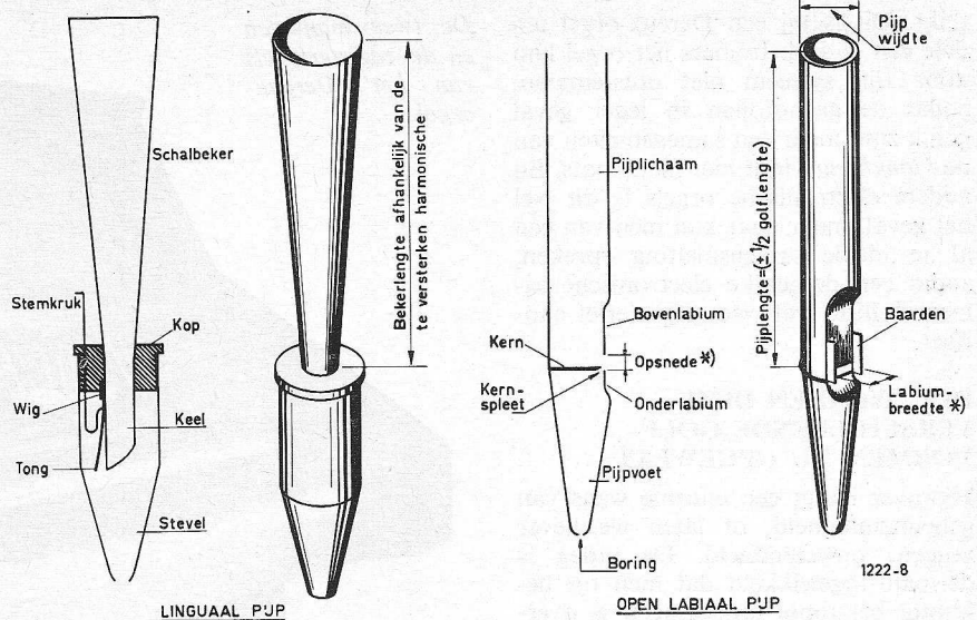
Figuur 6. Benamingen van de verschillende onderdelen van orgelpijpen. De pijpwijde, opsnede en labium-breedte zijn bepalend voor de klankkleur - de pijp-lengte voor de toonhoogte, in afwijking met de linguaalpijp waarbij de lengte en maat van de tong de toonhoogte bepaalt en de beker alleen maar wordt „afgestemd” op een bepaalde boventoon.
