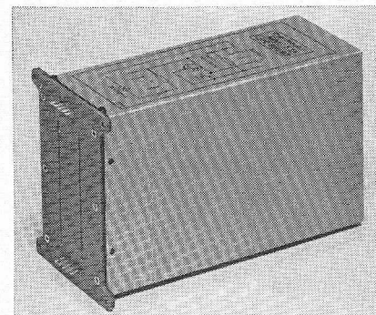
Ovenje voor het in temperatuur constant houden van 1 à 3 gedrukte schakelingen van max. 75 × 135 mm is ontwikkeld door Fuba (3202 Bad Salzdetfurth). Dit type ETA heeft een constantheid tot ± 0,1 °C bij 35 °C of 70 °C.
