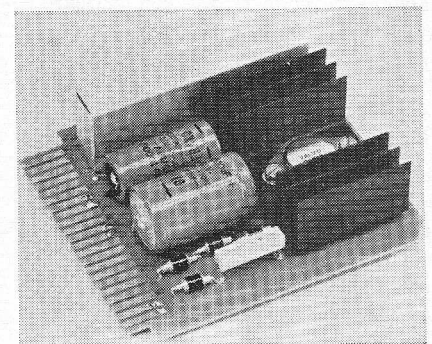
Stabilisatie-apparaat voor lage spanningen van Fuba (3202 Bad Salzdetfurth). Stabiliseert 4 laagspanningen van 6 en 18 volt bij 0,7 en 3 A nog bij hoge omgevingstemperaturen (tot 85 °C) dankzij toepassing van silicon transistoren en tantal-electrolytische condensatoren.
