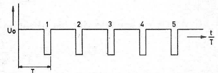
Figuur 2. Ingangsimpulsen voor de schakeling van figuur 1
